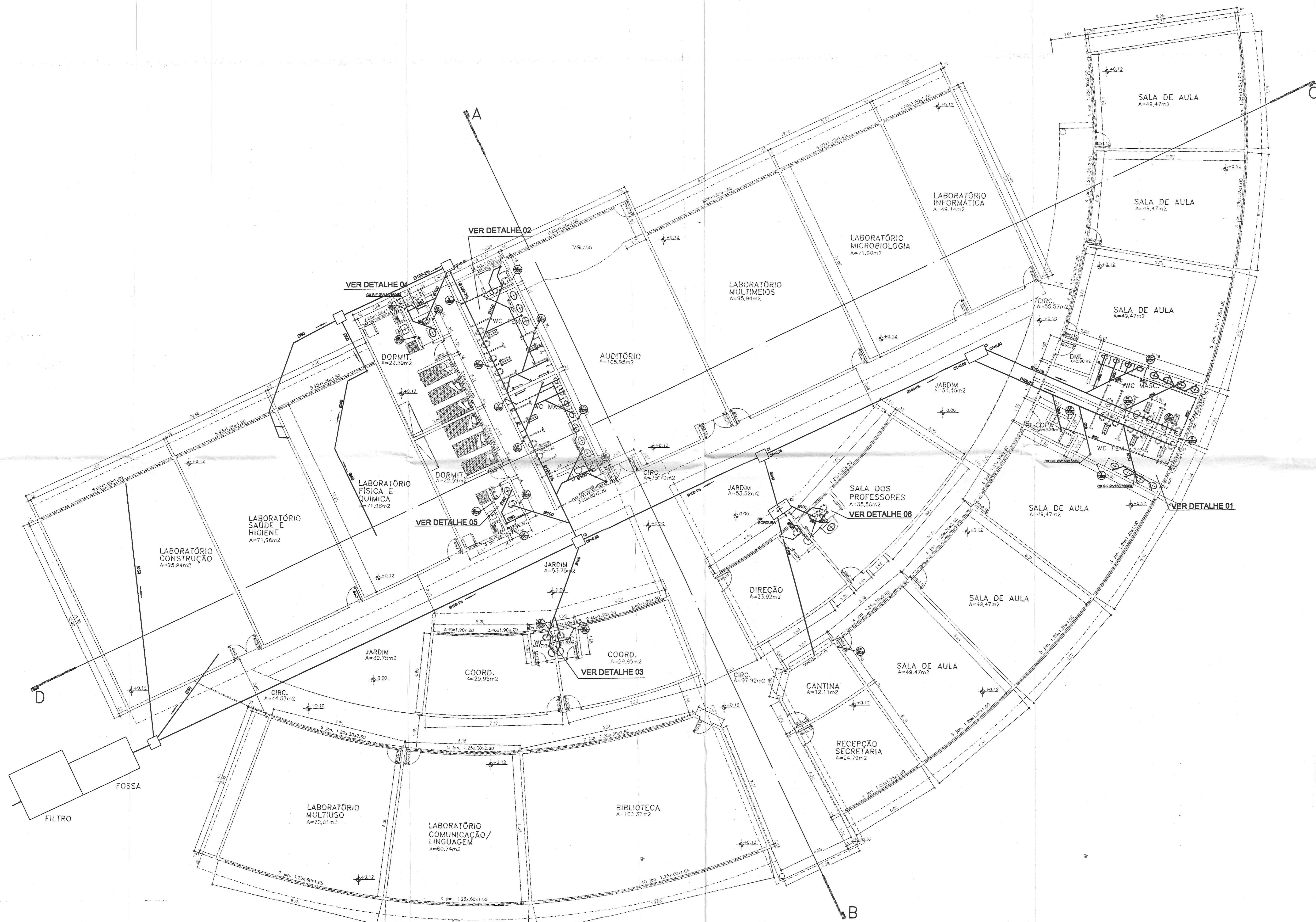
PLANTA BAIXA PAV. TÉRREO ESCALA 1:100
